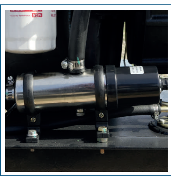
Precalentador
