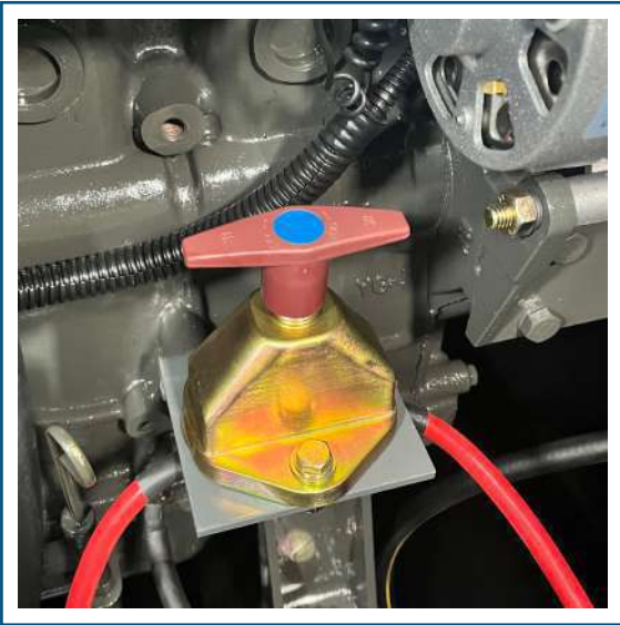
Cortacorriente
