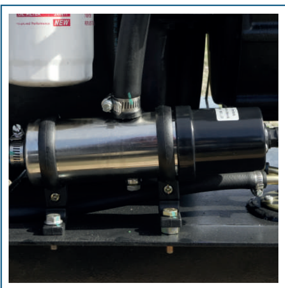
Precalentador
