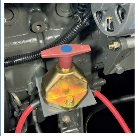
Cortacorriente
